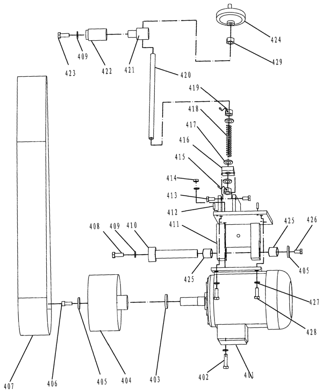
Рис. 16: Схема запасных частей 5
