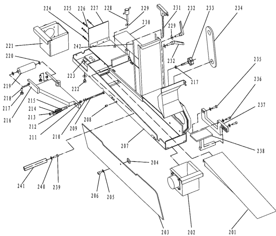
Рис. 14: Схема запасных частей 3
