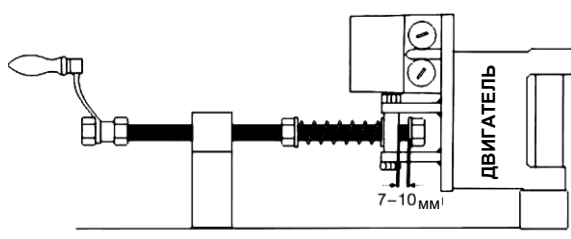
Рис. 7: Натяжка ремня.
