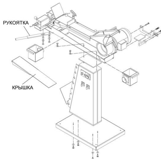
Рис. 4: Установка вырубного пресса для труб / ленточно-шлифовального станка.
