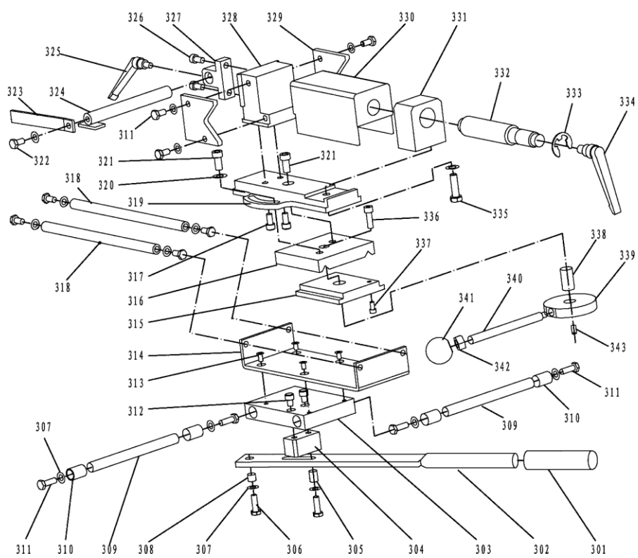
Рис. 15: Схема запасных частей 4
