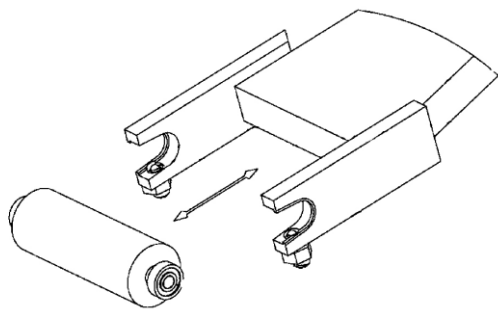
Рис. 6: Замена шлифовального валика.
