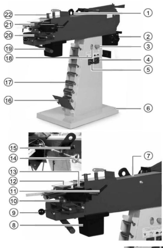
Рис. 3: Устройство станка
