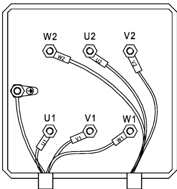
Рис. 5: Соединение двигателя
