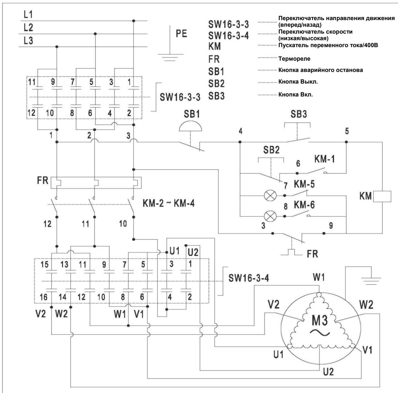
Рис. 17: Схема электрических соединений
